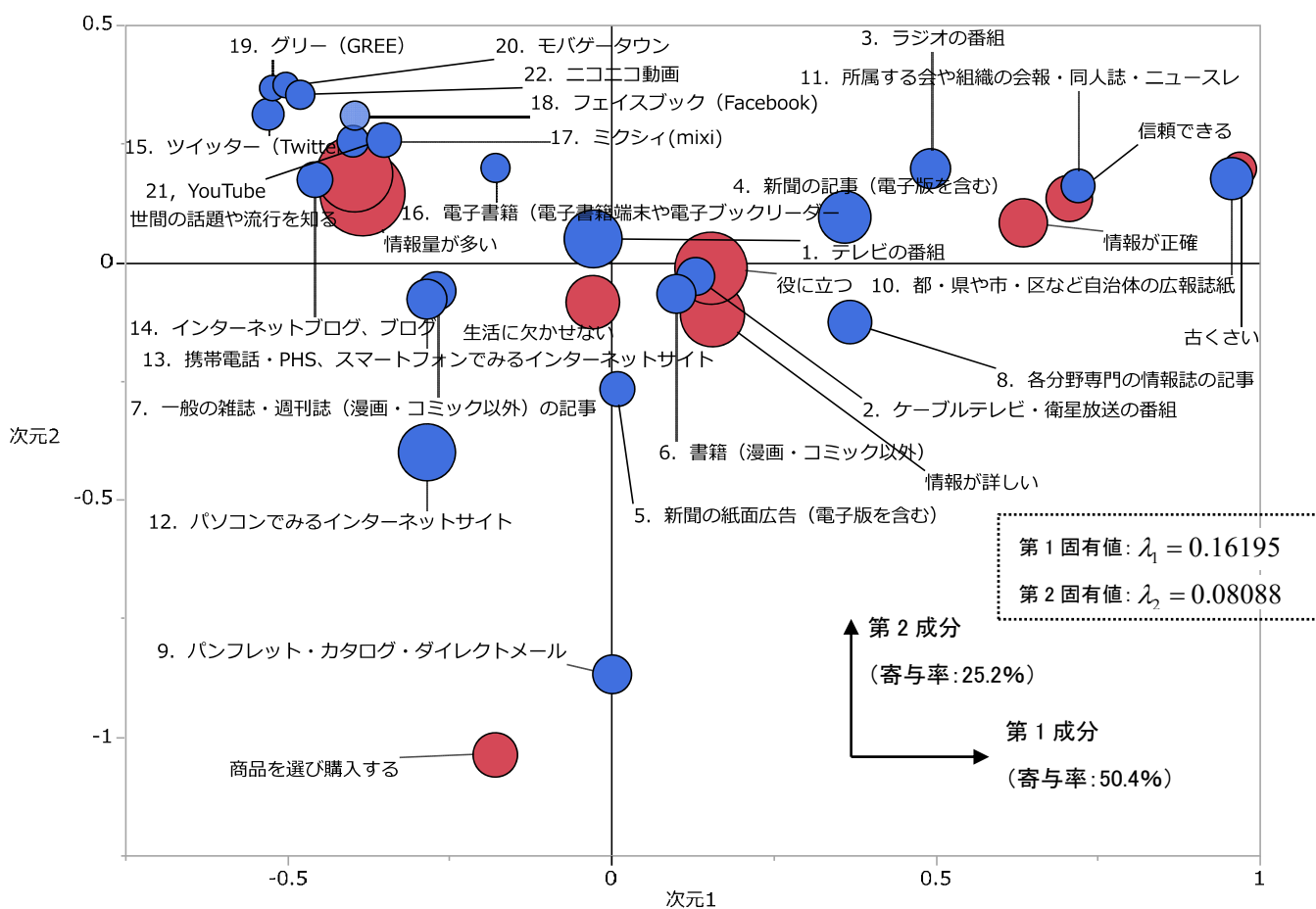
図 5 「情報源」と「評価項目」の同時布置図
