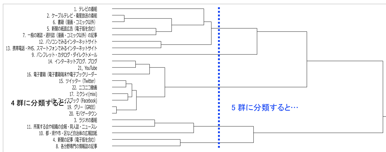
図 6 「情報源」の分類(デンドログラム)
