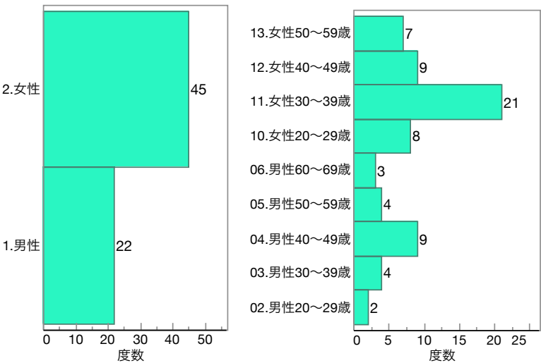
図 2 クラスター02 の性年齢区分の構成
