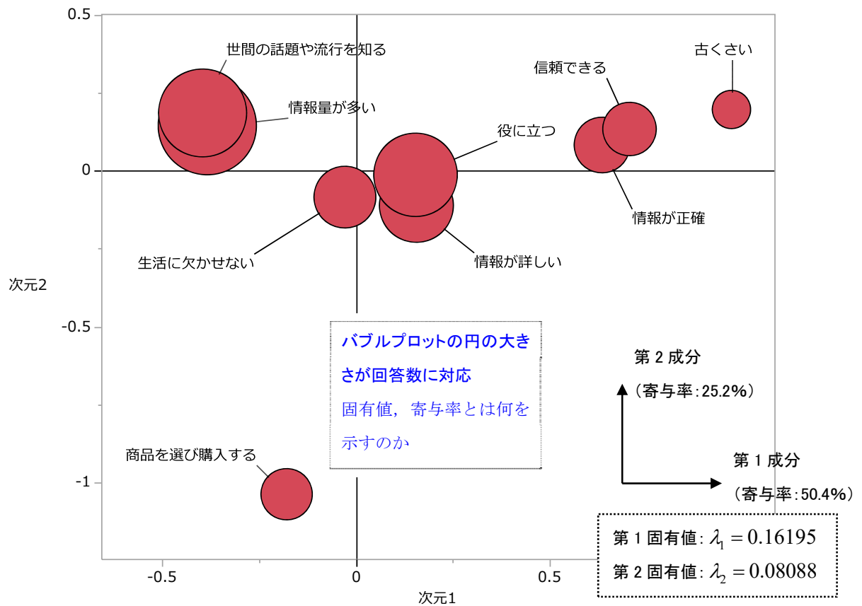
図3 「評価項目」の布置図(第1, 第2成分)
