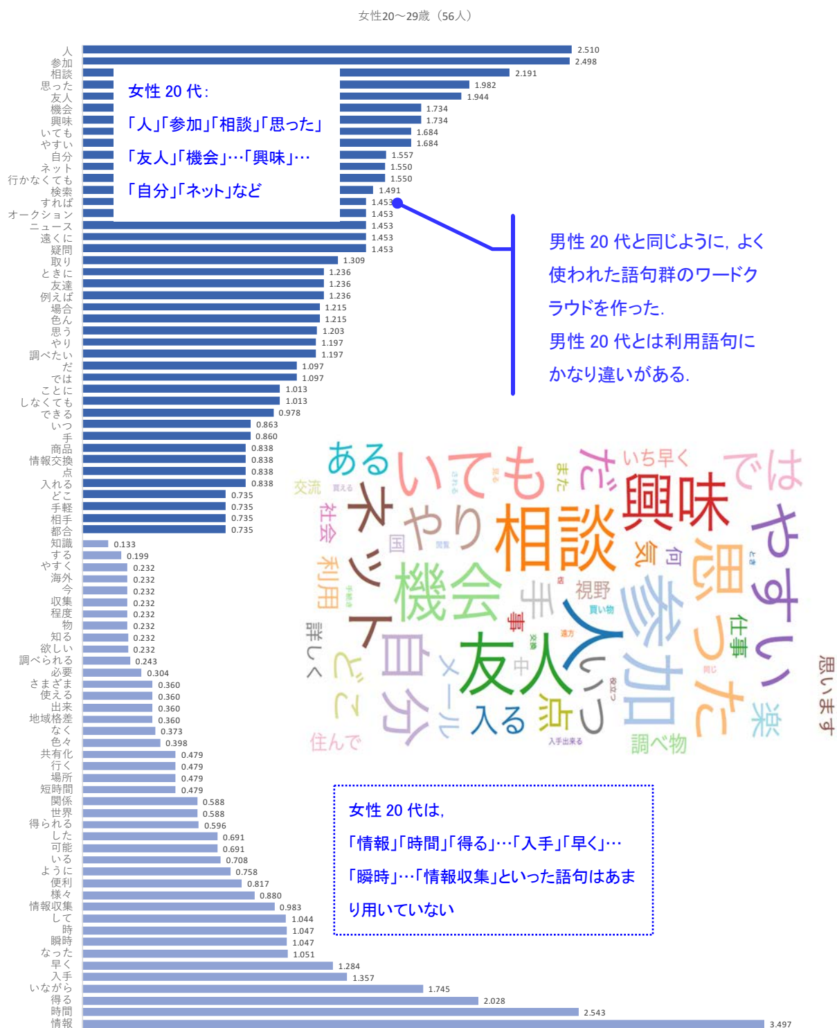
図 9 女性 20 代の語句群，検定値の特徴とワードクラウド
