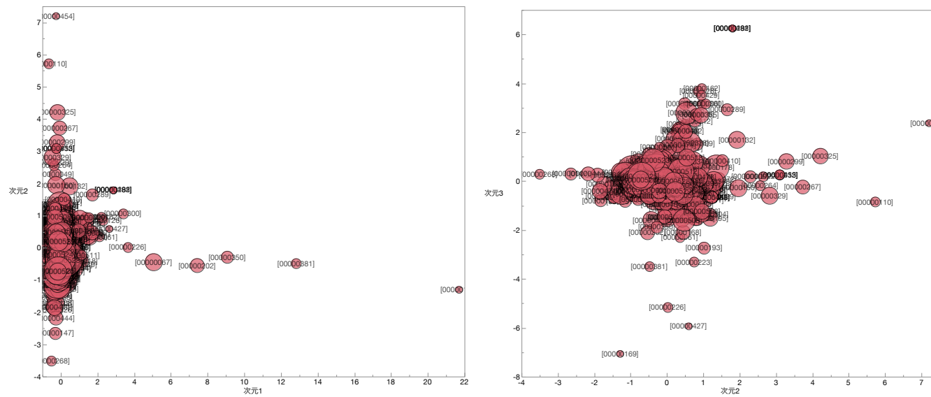
図 A2 対応分析で得た成分スコア
