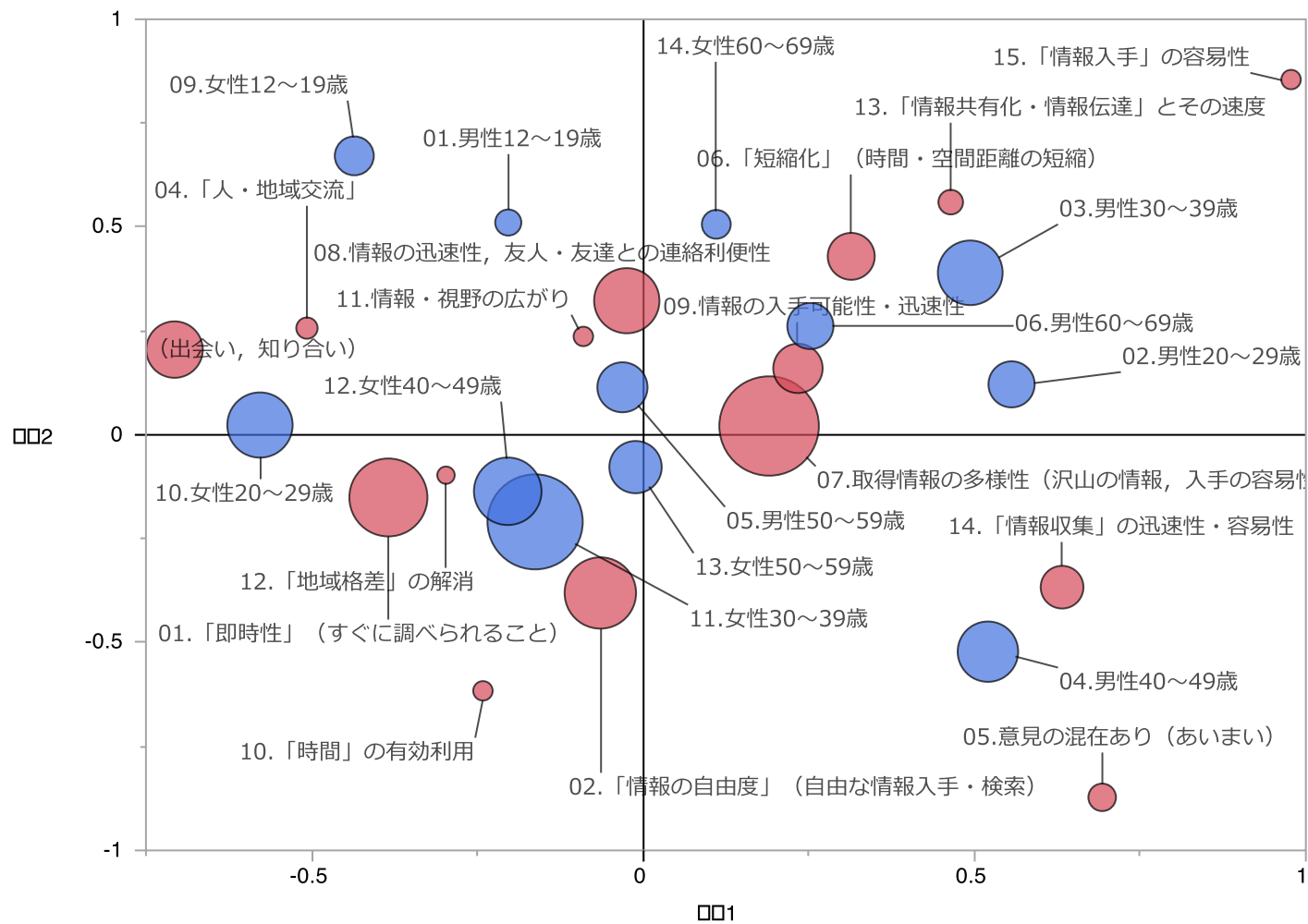
図 6 対応分析の結果 はじめの2成分(同時布置図)
