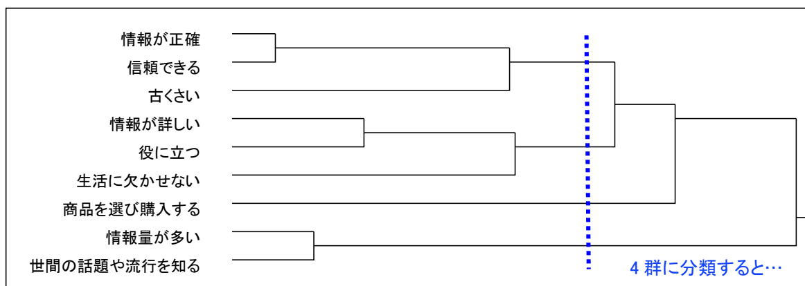
図 4 評価項目の分類(デンドログラム)
