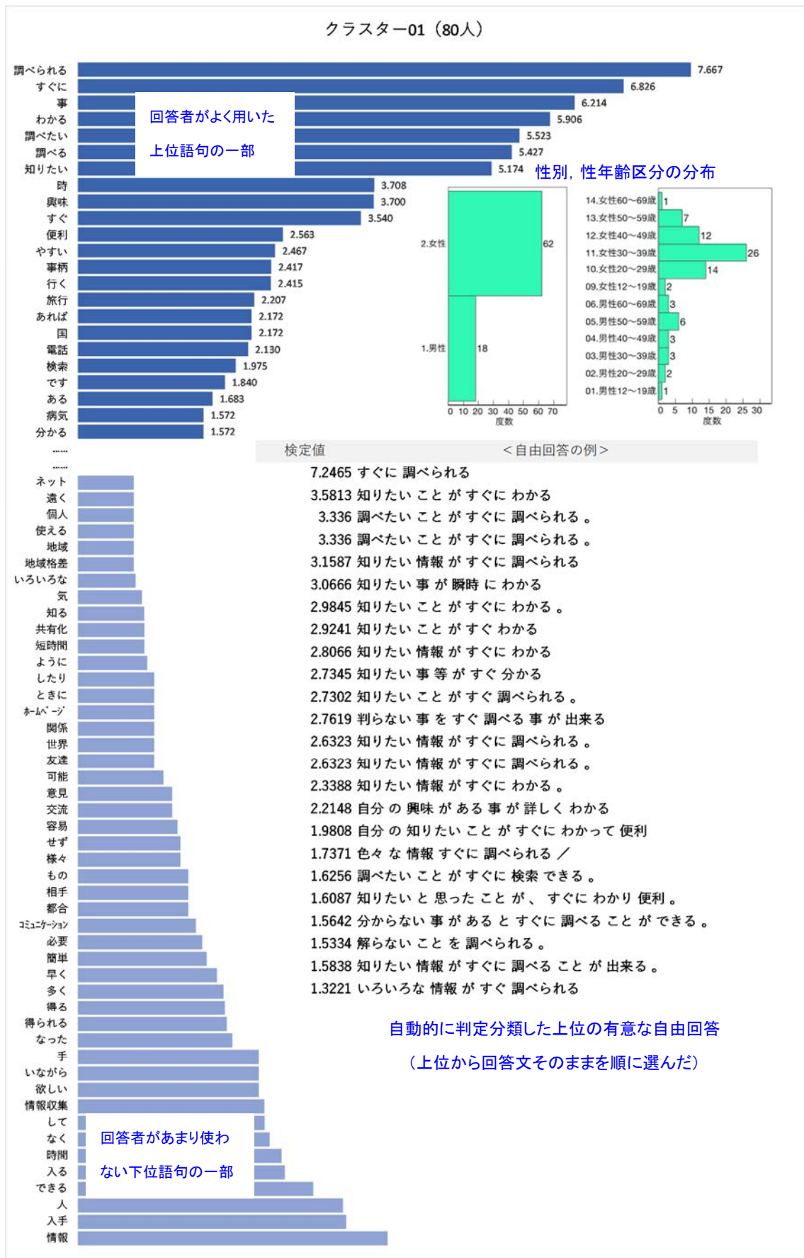
図 2 クラスター01 の基本情報
