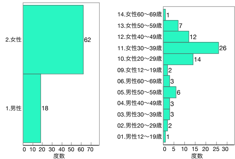
図 A3 クラスター01 の性年齢区分の構成
