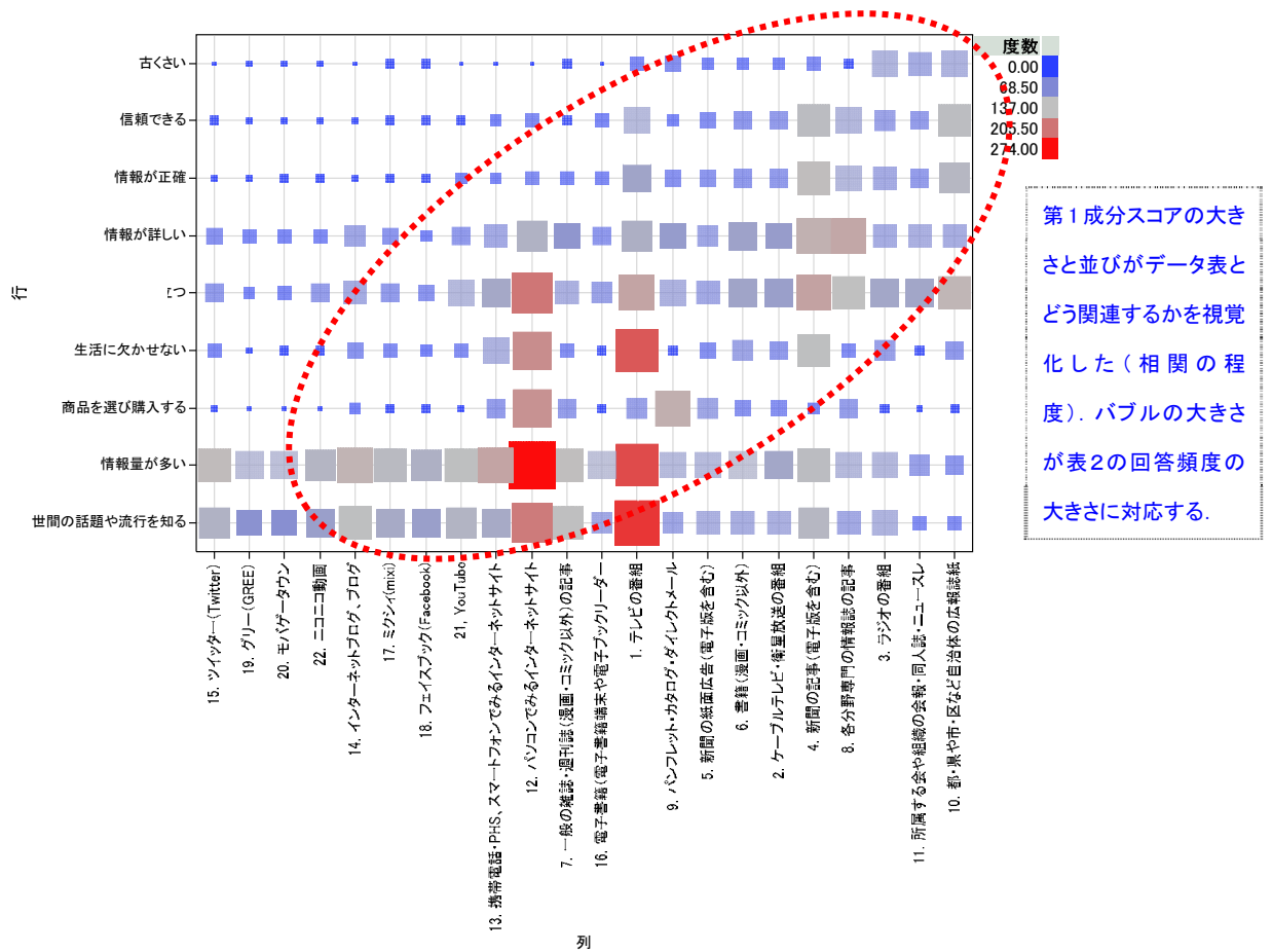
図2 データ表の特徴観察(第1成分スコアについて表2の行と列を並べ替え)
