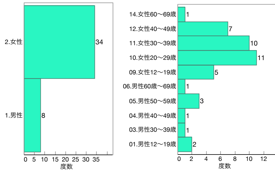
図 3 クラスター03 の性年齢区分の構成
