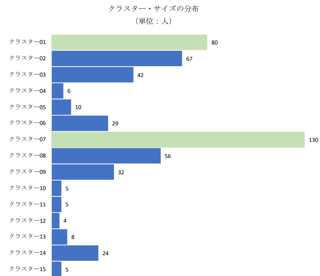
図 A1 回答者(503 人)の分類でえたクラスター・サイズの分布(*)サイズの大きい 2 つのクラスターの色を変えてある.
