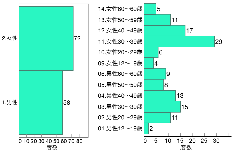
図 4 クラスター07 の性年齢区分の構成
