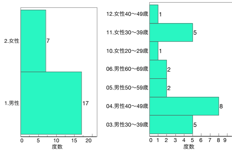
図 A クラスター14の性年齢区分の構成
